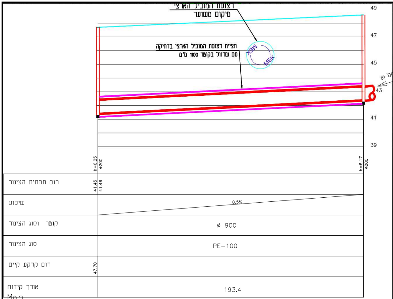
איור 3 – חתך לאורך הקידוח האופקי
