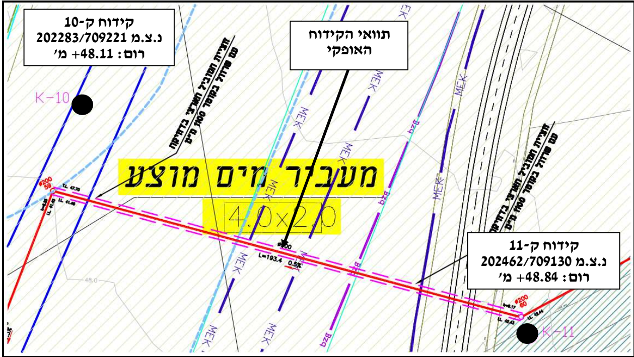
איור 2 – תכנית כללית של הקידוח האופקי
