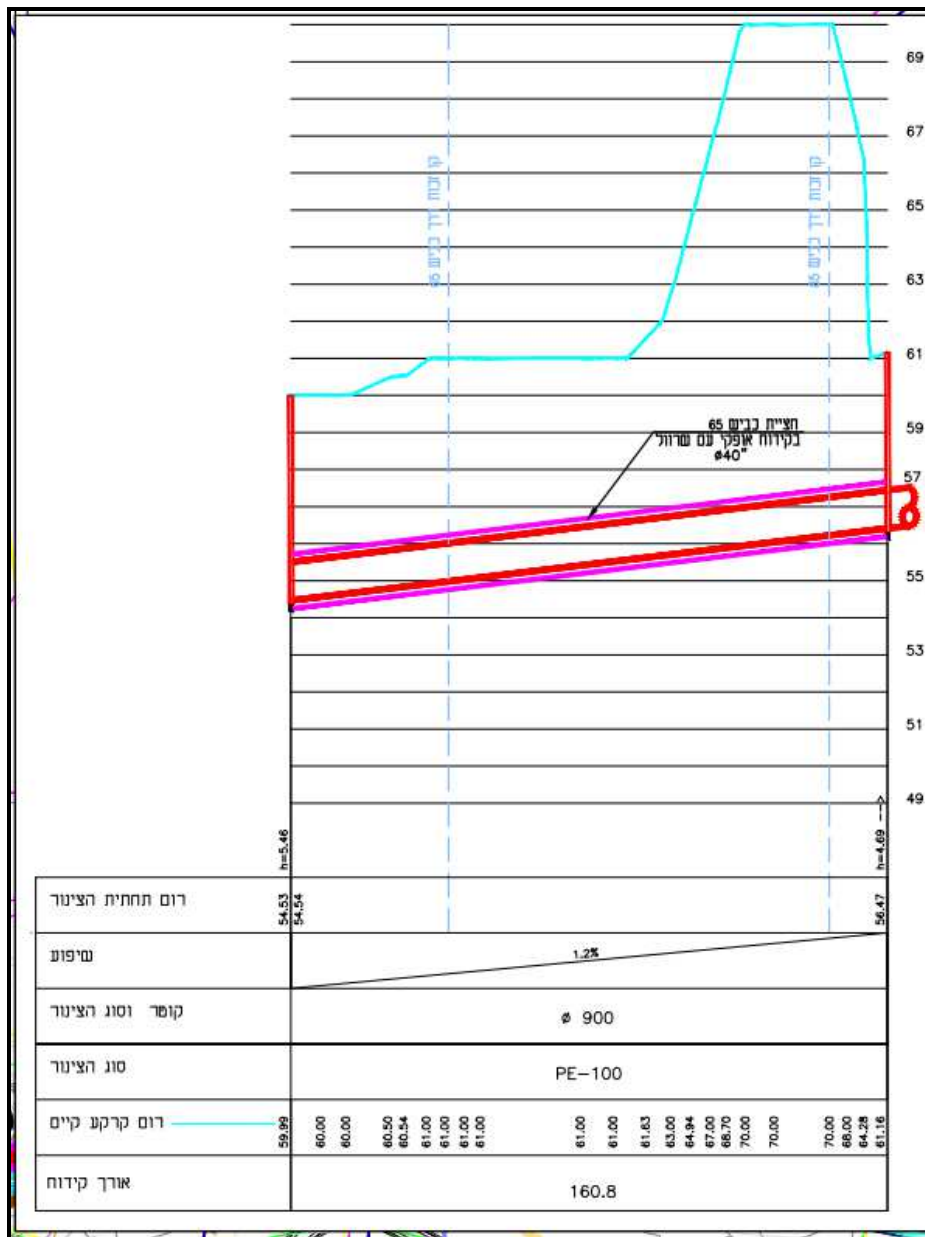
איור 3 – חתך לאורך הקידוח האופקי
