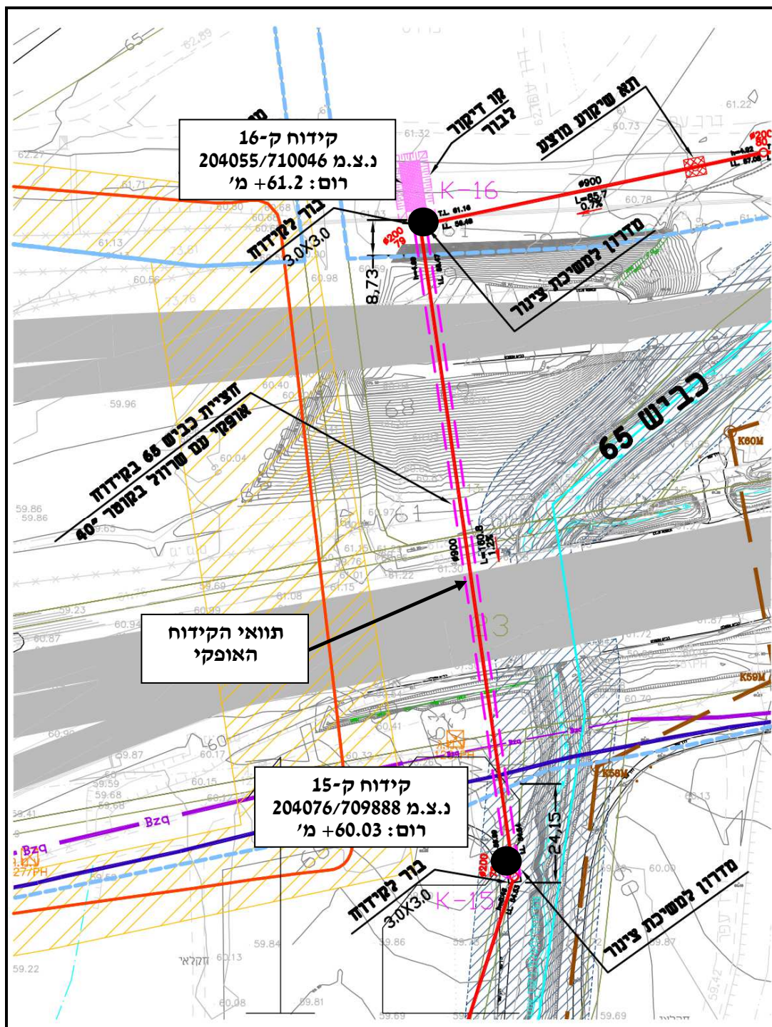
איור 2 – תכנית כללית של הקידוח האופקי
